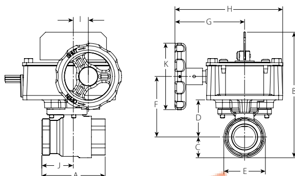
ROSCADO X ROSCADO
