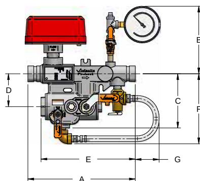
Tamaños nominales de 1 ¼ – 2 ½/32 – 50 mm
