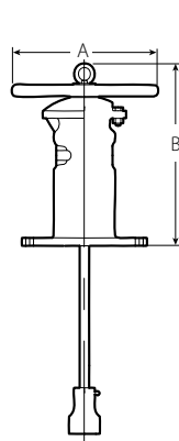
POSTE INDICADOR DE PARED SERIE 773
