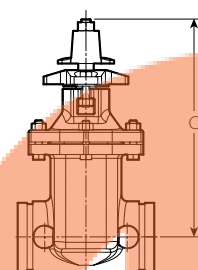
LÍNEA CENTRAL DE LA VÁLVULA DE COMPUERTA NRS (SE MUESTRA SERIE 772H)
