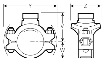
Salida ranurada
