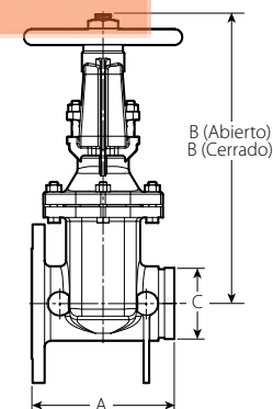
VÁLVULA DE COMPUERTA SERIE 771F OS & Y
